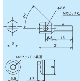
AT-N2 注記1) 寸法公差±0.5
