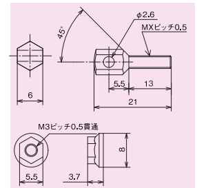
AT-N2 注記1) 指定以外の寸法公差 ±1.0
