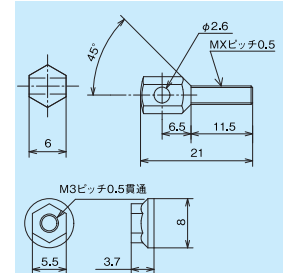
AT-N12 注記1) 寸法公差±0.5
