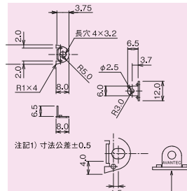
AT-04R 注記1) 寸法公差±0.5
