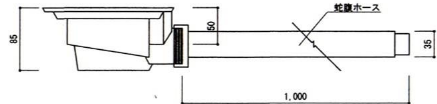
排水トラップ S=1/5
