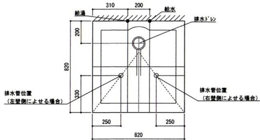
床平面図
