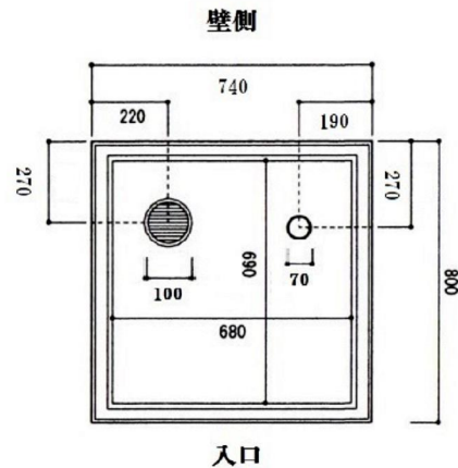
天井詳細図 =1/20
