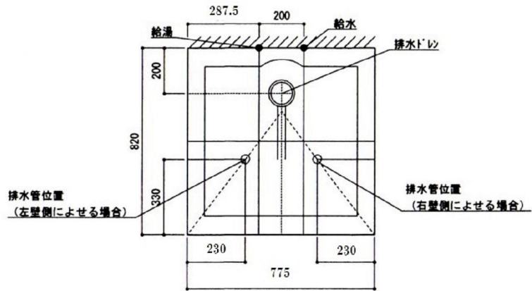
床平面図
