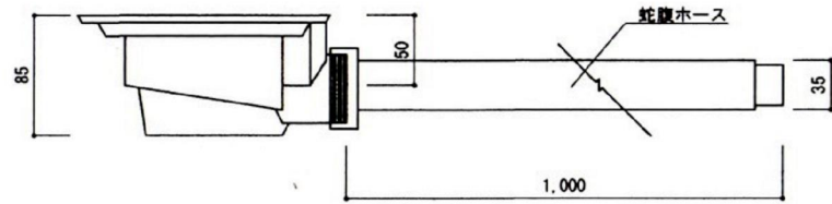
排水トラップ S=1/5
