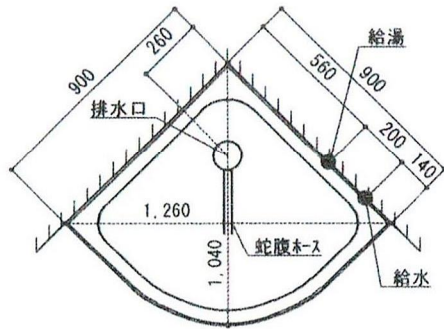
床平面図
