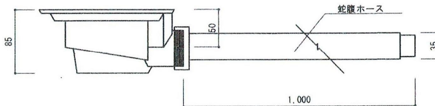
排水トラップ S=1/5
